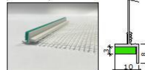
Profilo con rete per rasatura per cappotto esterno (non garantita per interno)
