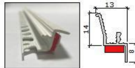
Profilo per intonaco interno con asole
