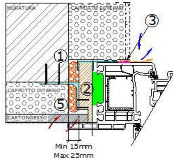
CONTROTELAIO STD LEGNO-ALLUMINIO Scasso e cartongesso interno Profilo prefinito per finiture esterne
