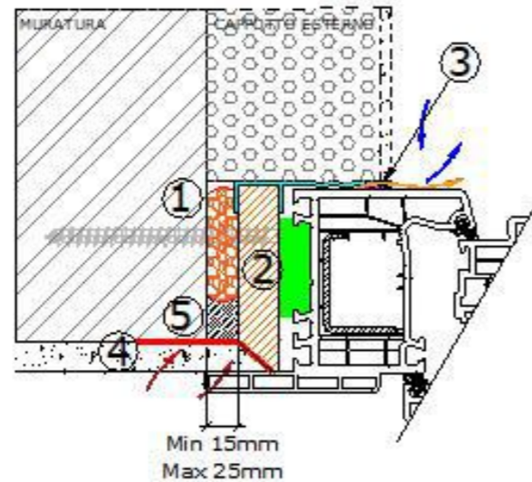
CONTROTELAIO STD LEGNO-ALLUMINIO Barriera vapore interna Profilo prefinito per finiture esterne
