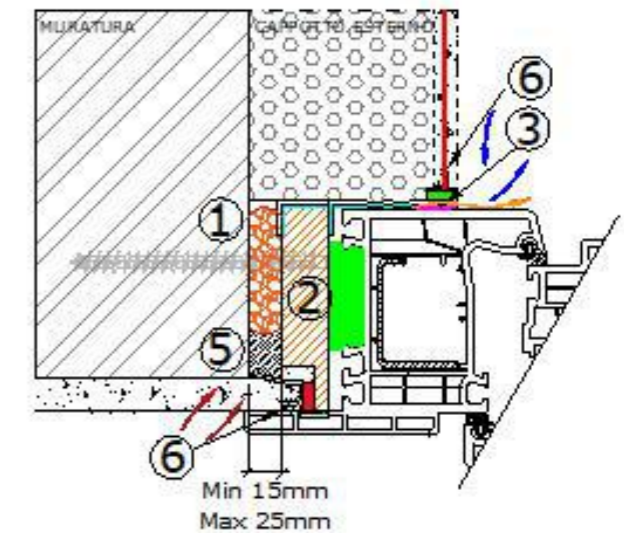
CONTROTELAIO STD LEGNO-ALLUMINIO Profilo interno con asole per intonaco Profilo esterno con rete per cappotto
