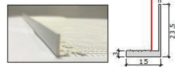
Profilo con rete per rasatura per cappotto esterno (non garantita per interno)
