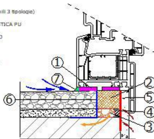
CONTROTELAIO STD LEGNO-ALLUMINIO TRAVERSO INFERIORE sezione laterale
