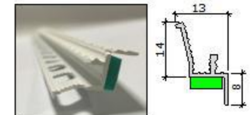
Profilo per con asole intonaco esterno
